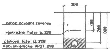
ULOŽENÍ KABELU NN
