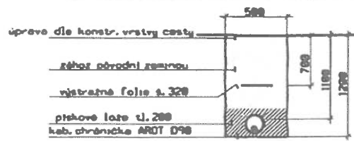
ULOŽENÍ KABELU NN V CESTĚ - PŘEKOP
