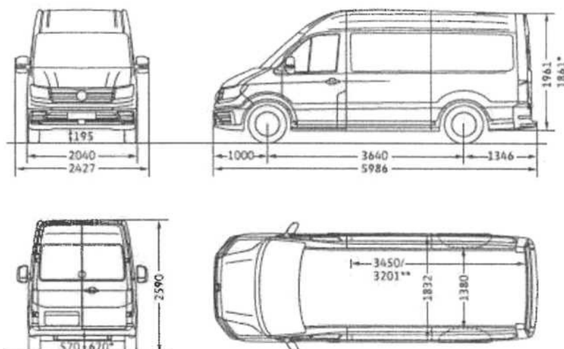
Crafter 30/35 skříňový vůz střední rozvor s vysokou stěchou
