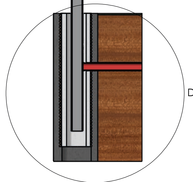
ŘEZ C-C MĚŘITKO 1 : 15
