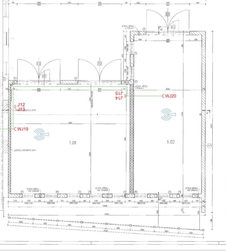
PŮDORYS 1.NP
