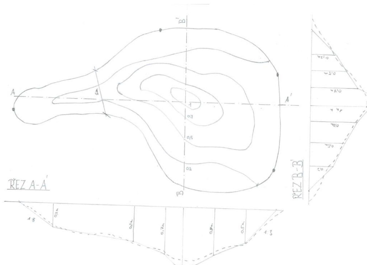
Příloha č. 5: Vzorový výkres a řez tůně
