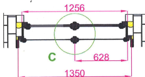
ŘEZ - PŮDORYS
