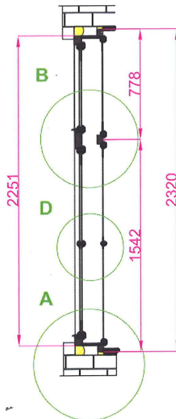
ŘEZ - BOKORYS
