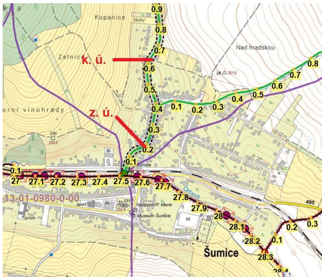
Příloha č. 1: Situace budoucího staveniště
