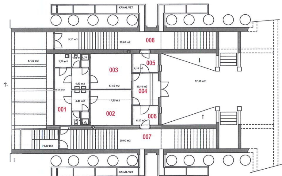
1 SUTERÉN -3,000
