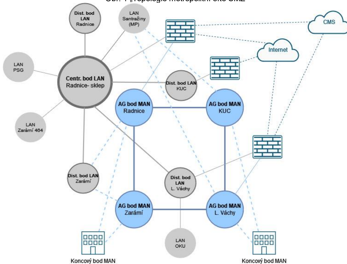
Obr. 1 „Topologie metropolitní sítě SMZ“
