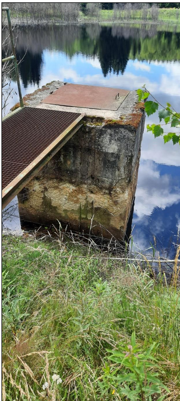
Obrázek 5 - pohled na špatný technický stav požeráku.
