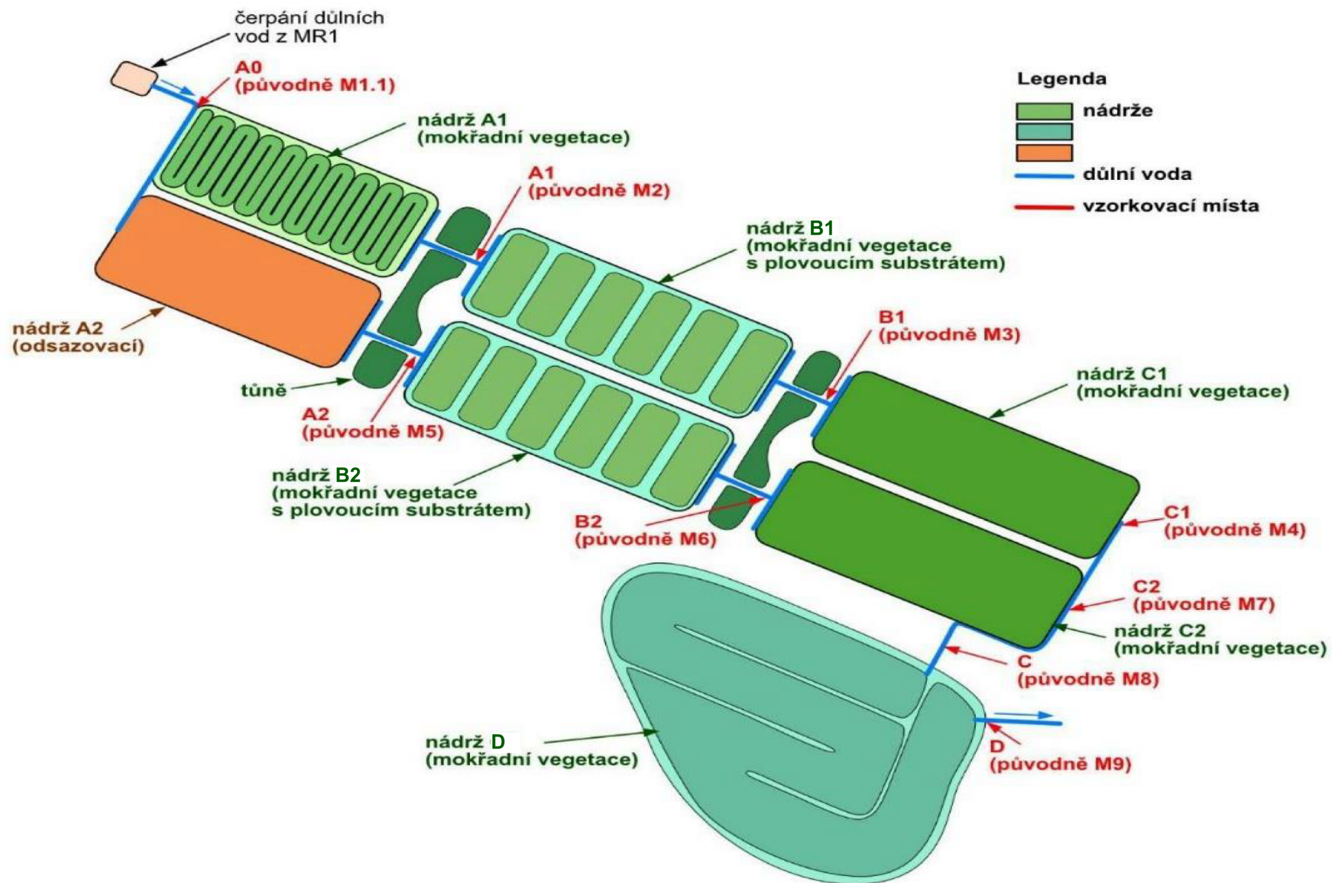
Obr. 1 Schéma Biotechnologického systému čištění důlních vod z MR1 podle návrhu firmy Terén Design, s.r.o. s vyznačením jeho jednotlivých částí.
