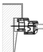
Začištění Rekord typ B
