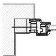
Špaletové začištění typ A1
