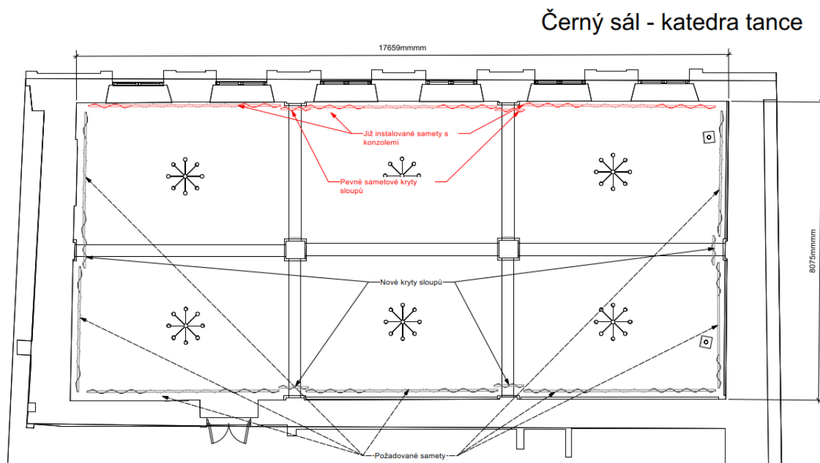
Obrázek 1 – Dispozice sametů
