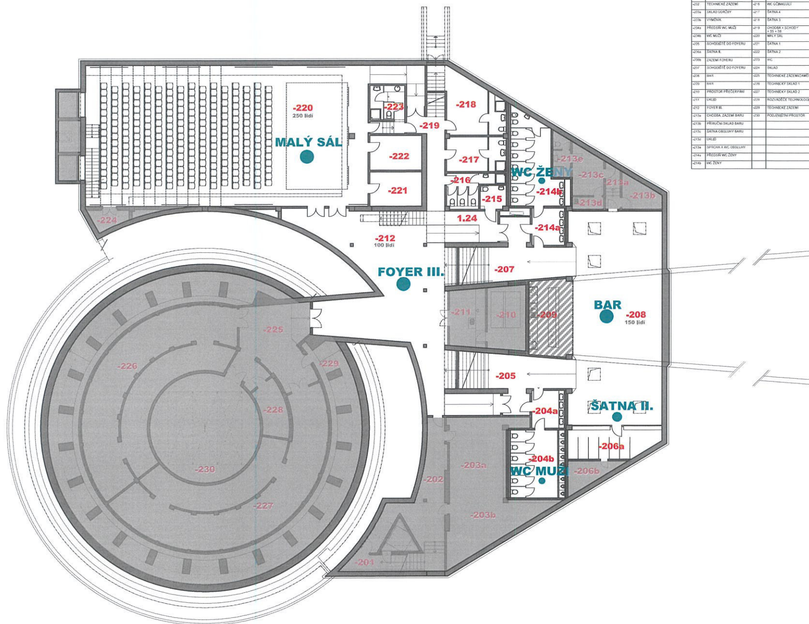
TABULKA MÍSTNOSTÍ 2PP-2P1
