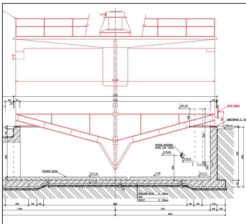
Schéma nádrže
