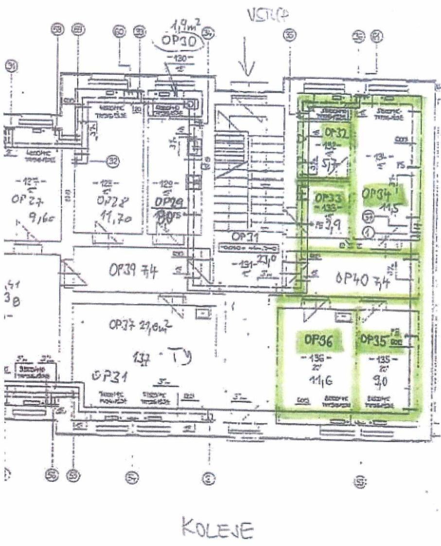
Příloha č. 1 – Půdorys objektu výpravní budovy Horní Lideč
