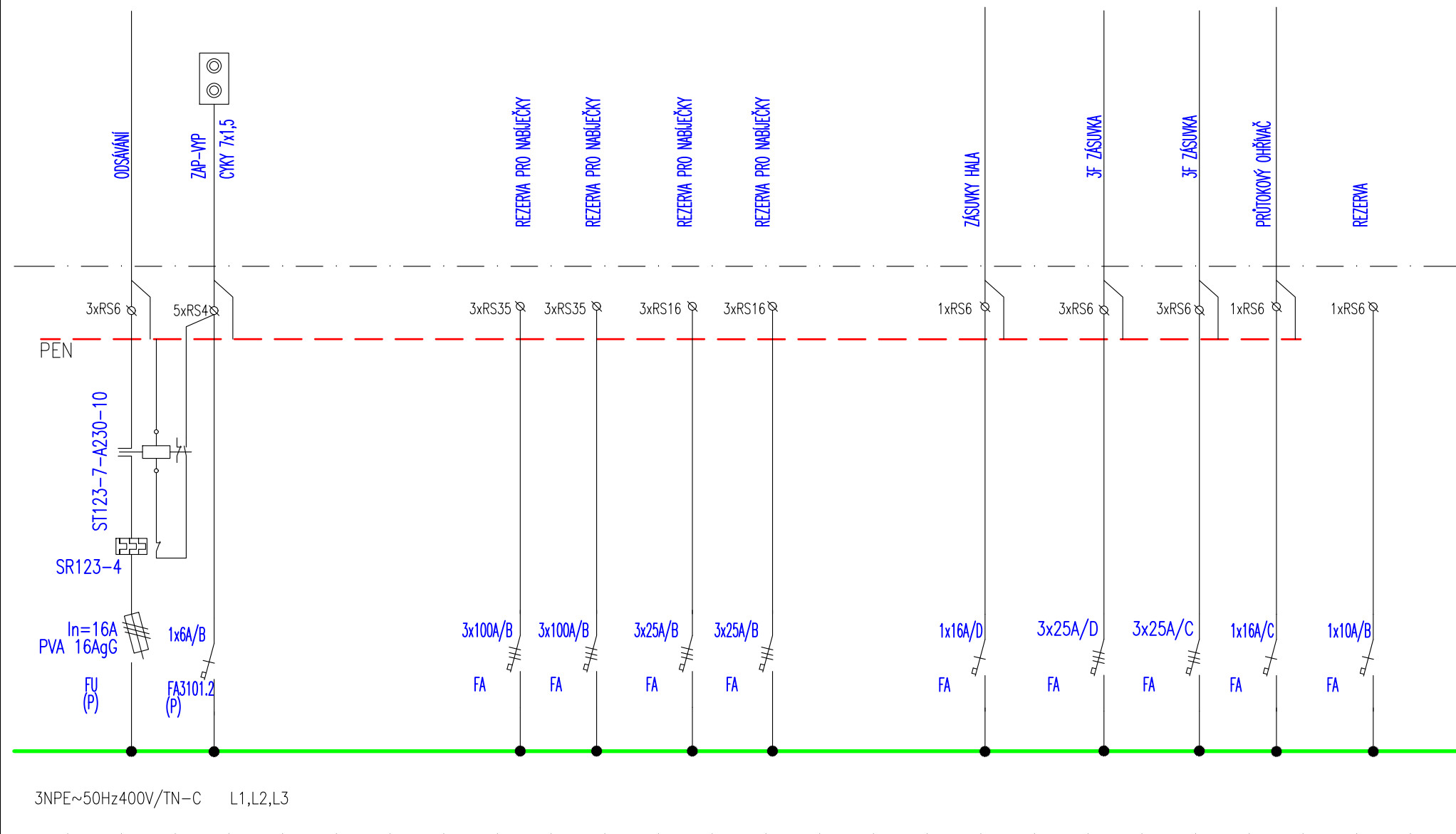
Rozvaděč RN2
