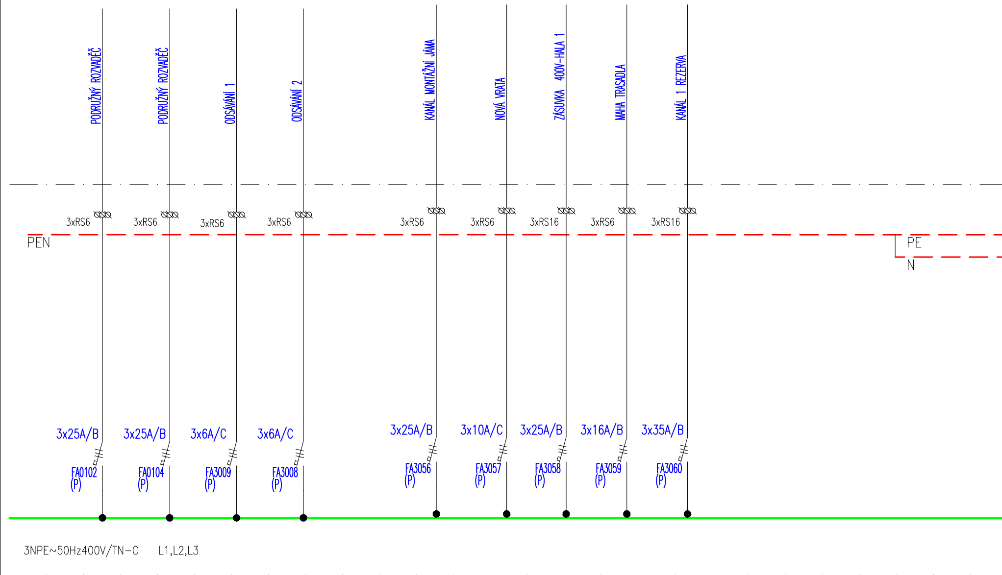
Rozvaděč RN1 RM1
