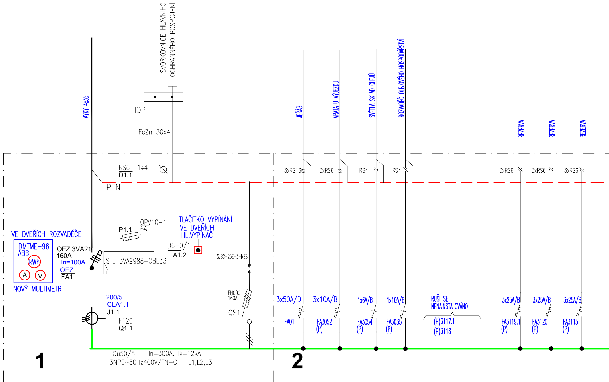
Rozvaděč RN2
