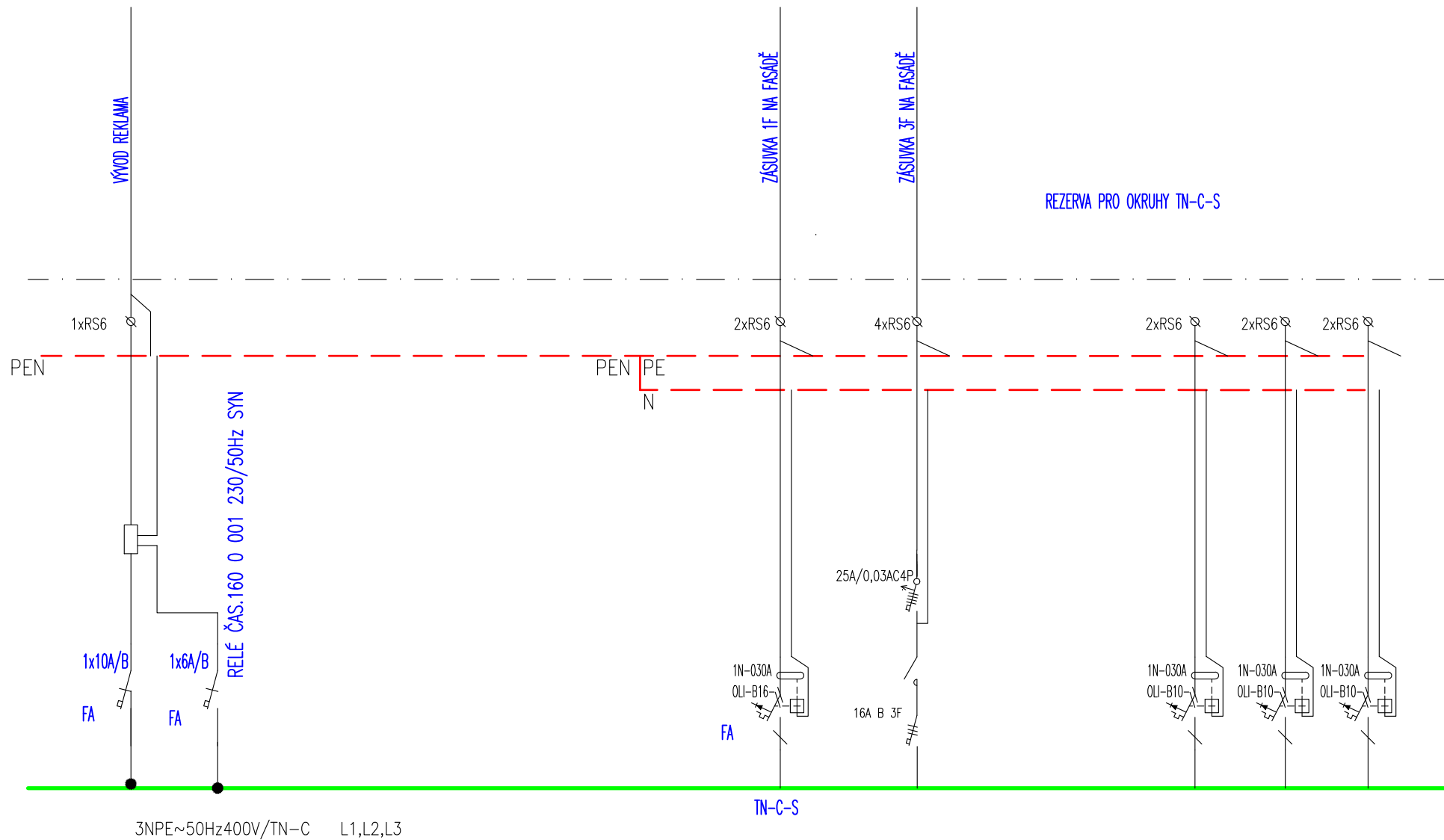
Rozvaděč RN2
