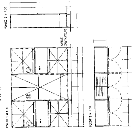
I. Sestava – 1x skříň vysoká satní h 1400mm, 2x skříň vysoká polcová s nikou h 1400mm 2400x1200x1820
