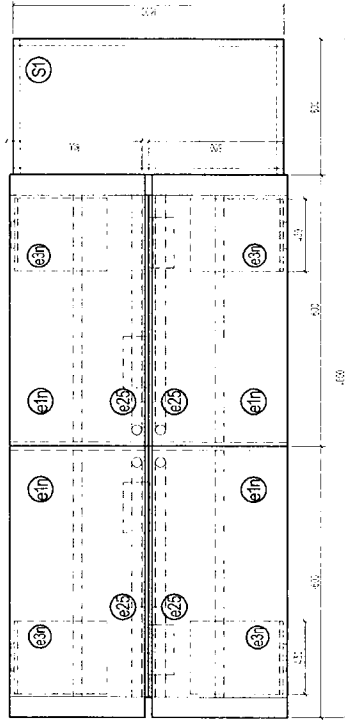
POHLED HORNÍ
