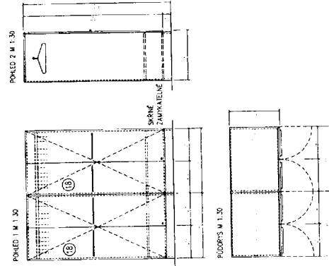
III. Sestava – 2x skříň vysoká satní h 1600mm 1600x1200x1820
