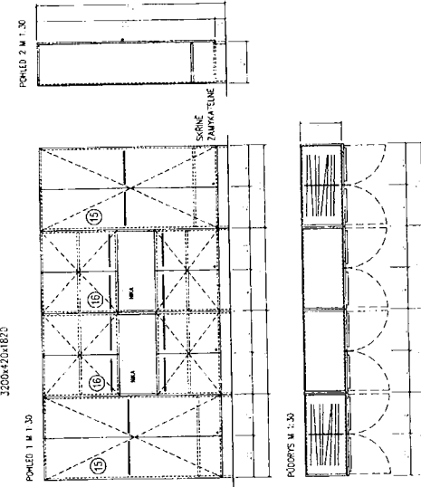
II. Sestava – 2x skříň vysoká satní h 1400mm, 2x skříň vysoká polcová s nikou h 1400mm 1200x1200x1820
