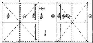
SKŘIN VYSOKÁ PŮLCOVÁ S NIKOU H: 400mm 800x420x1820
