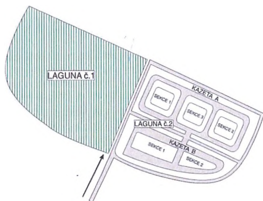
Obrázek č.1 – schematické naznačení rozmístění sekcí a kazet na laguně č.2
