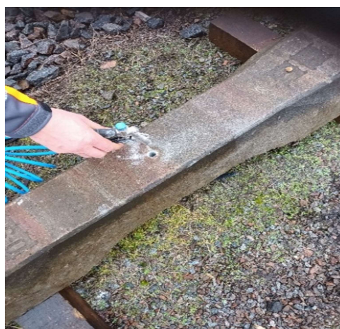
Obrázek 5 - Čištění otvoru
