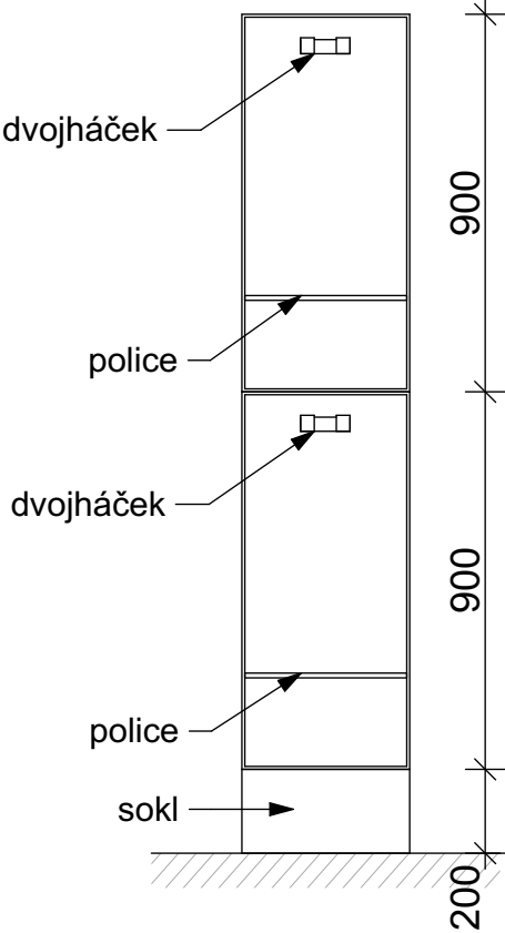
schéma umístění a opláštění skříněk
