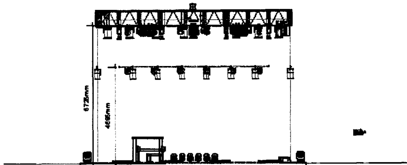
2 Front view Scale: 1:100
