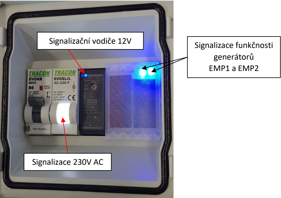
Obrázek SEQ Obrázok \* ARABIC 2 Rozvaděč, světelné kontrolky
