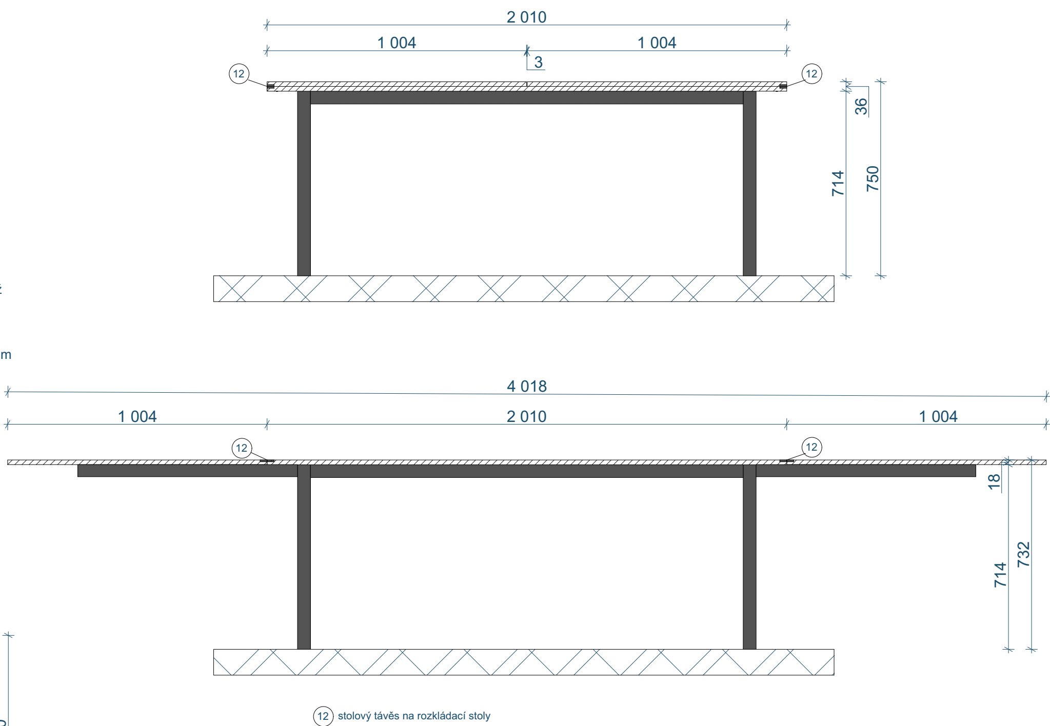
18 - Rozkládací stůl
