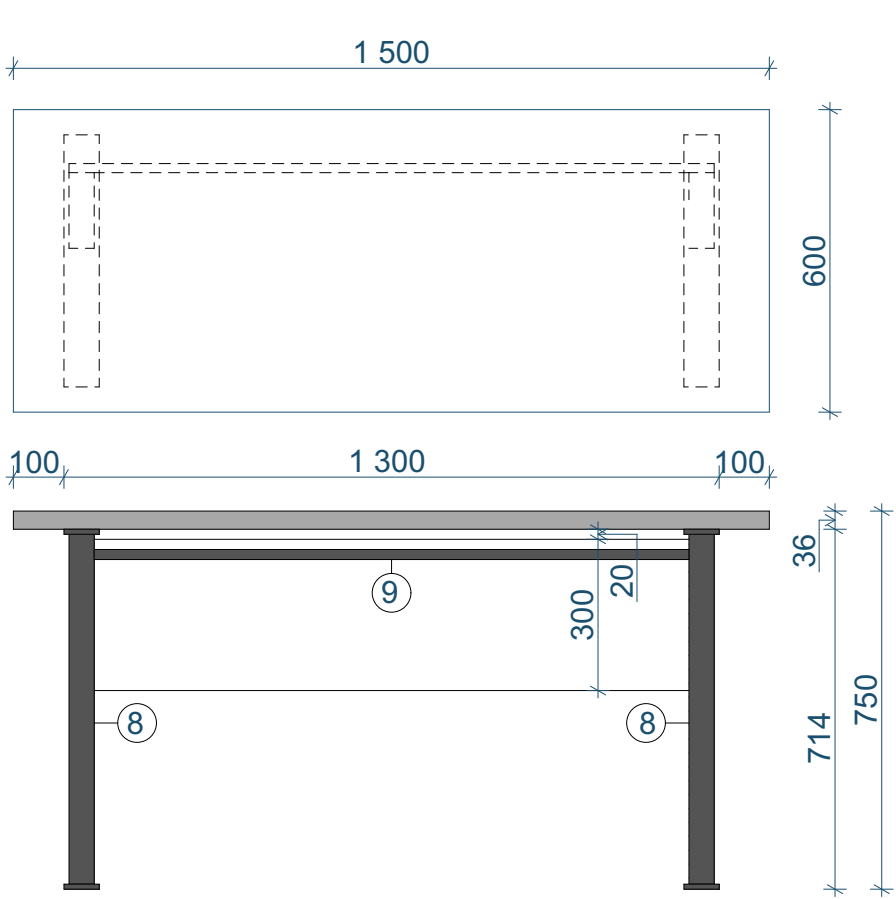
9 - Kancelářský stůl
