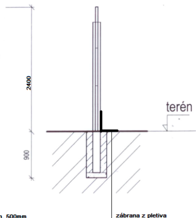
PŘÍČNÝ ŘEZ
