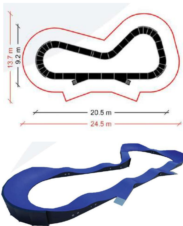
Schéma a rozměrové parametry sestavy
