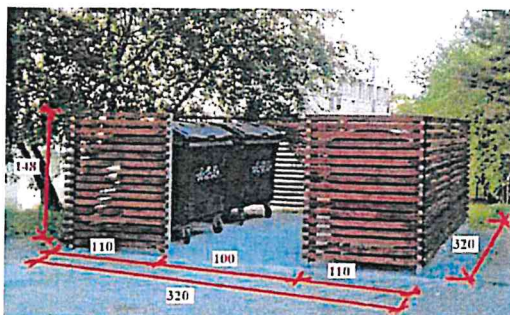
Obr. Kóje na popelnice – požadované řešení
