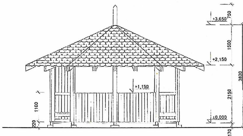
POHLED 1:50
