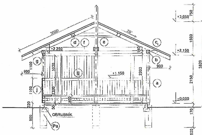
ŘEZ A 1:50
