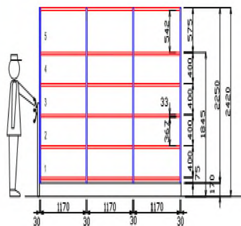
VÝŠKOVÉ ČLENĚNÍ POSUVNÉHO REGÁLU M1-M40
