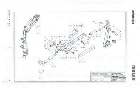
hlavní rameno 1
