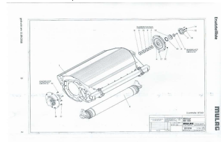
kopírovací válec
