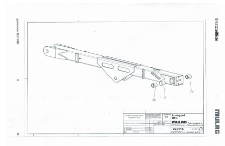
hlavní rameno 2
