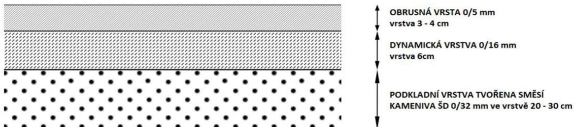
SKLADBA VRSTEV PRO POKLÁDKU MLATOVÉHO POVRCHU DLE METODIKY FLL
