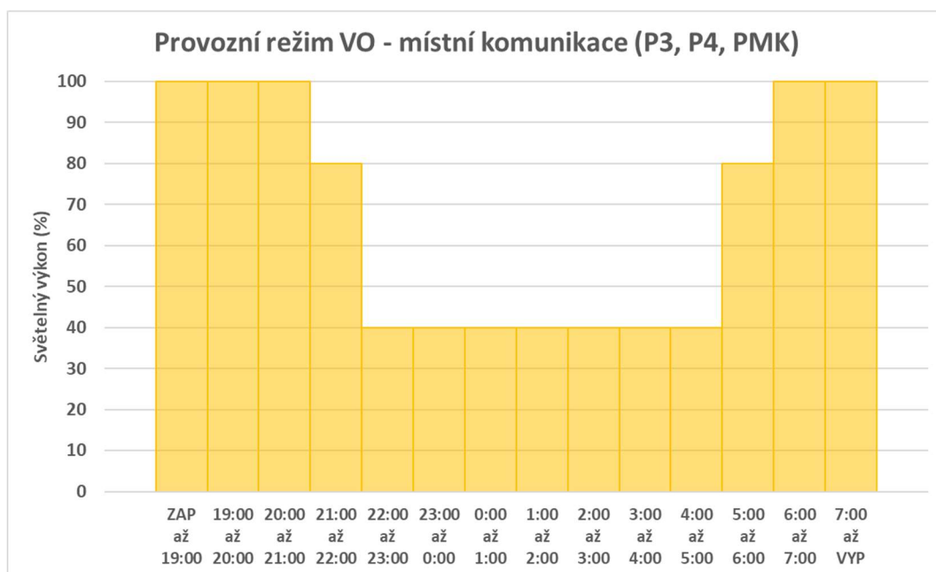
Graf 5 - Provozní režim VO – místní komunikace (P3, P4, PMK)
