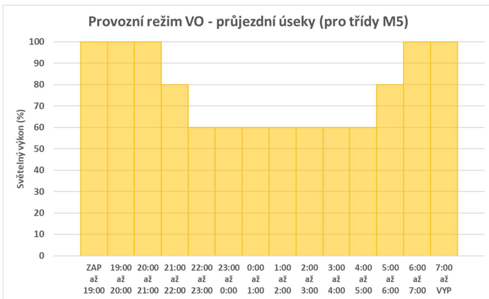
Graf 4 – Provozní režim veřejného osvětlení – Průjezdni úseky silnic s třídou osvětlení M5
