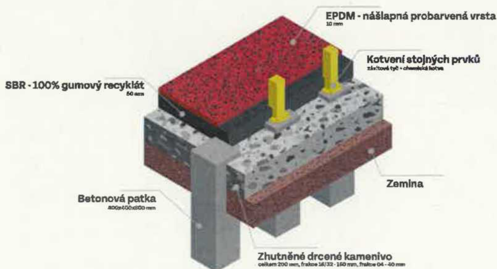
Řez spodní stavby s dopadovou plochou.
