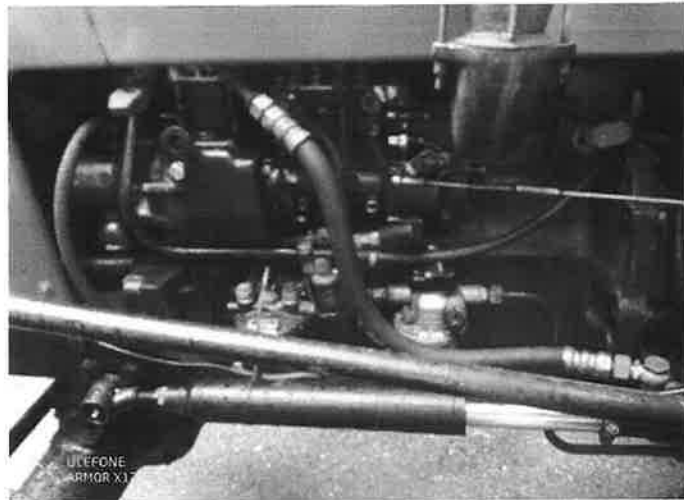
obr.4 - levý pohled (detail: motor 70HP)
