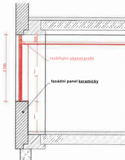
AD Řez A5 1:50
