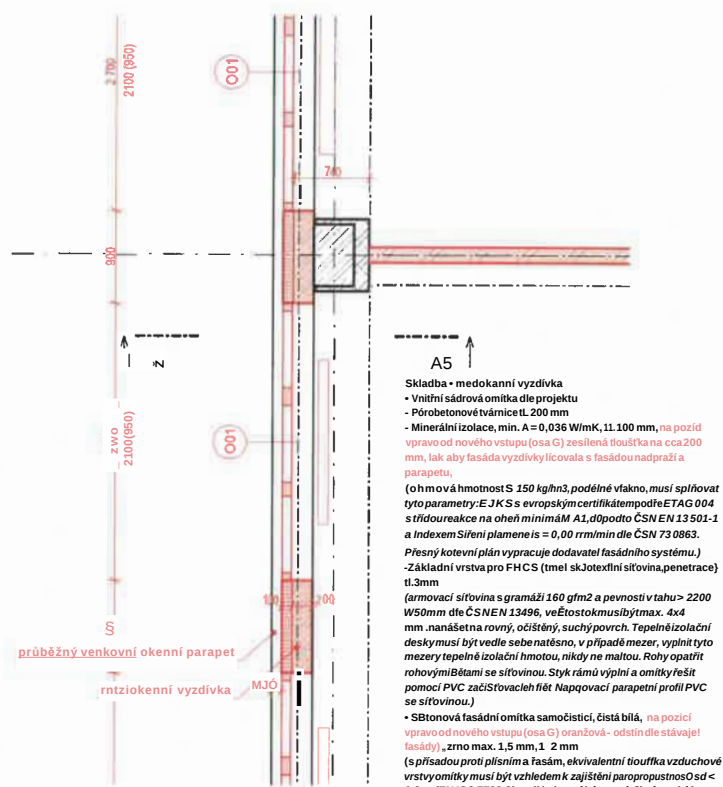
AD 1.NP okna nové 1:50
