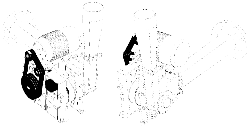
Obrázek 1: Reverzní vodní turbína včetně příslušenství.
