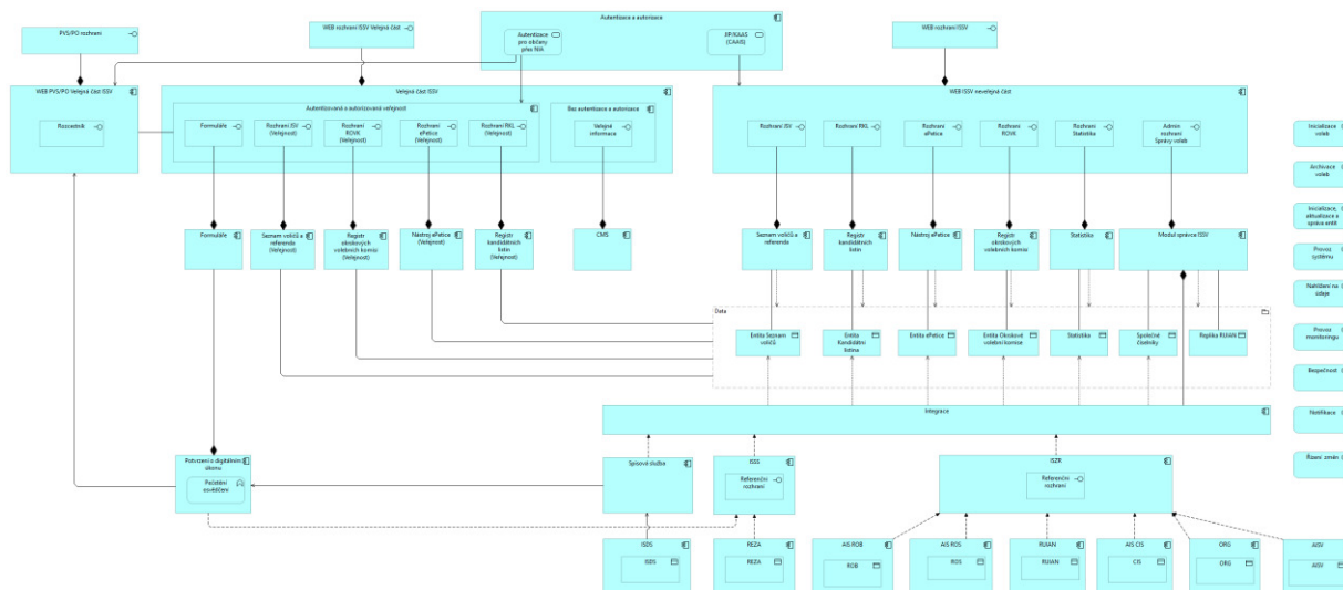
Schéma: Aplikační architektura
