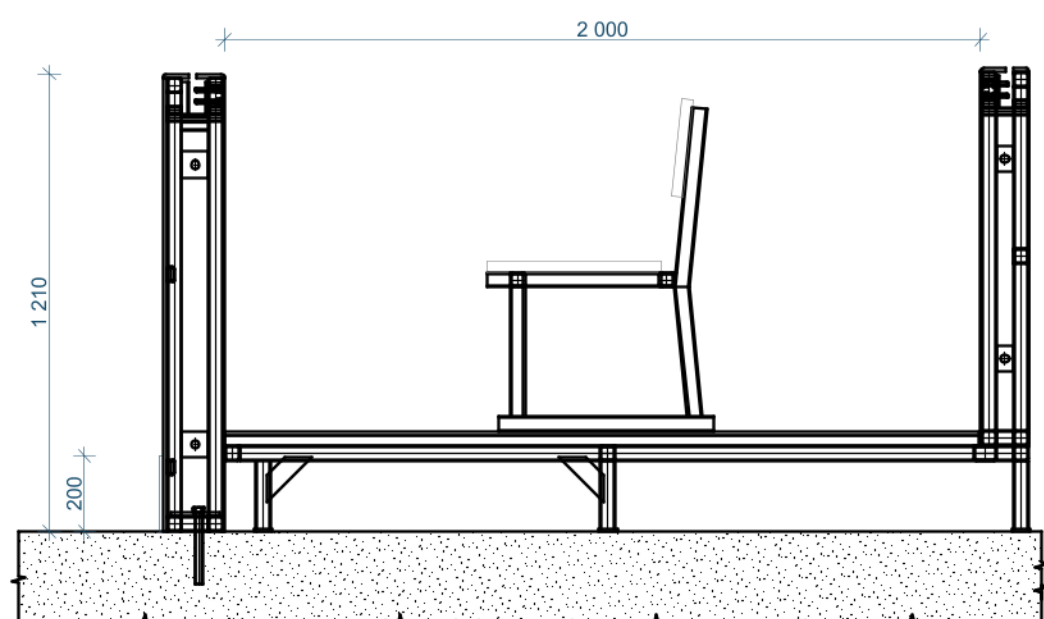
ŘEZ STŘÍDAČKOU M 1:20
