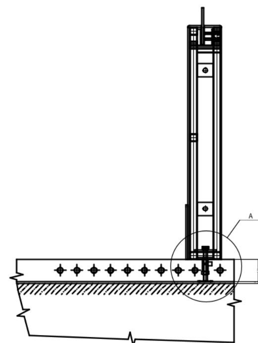
ŘEZ KOTVENÍ MANTINELU M 1:20
