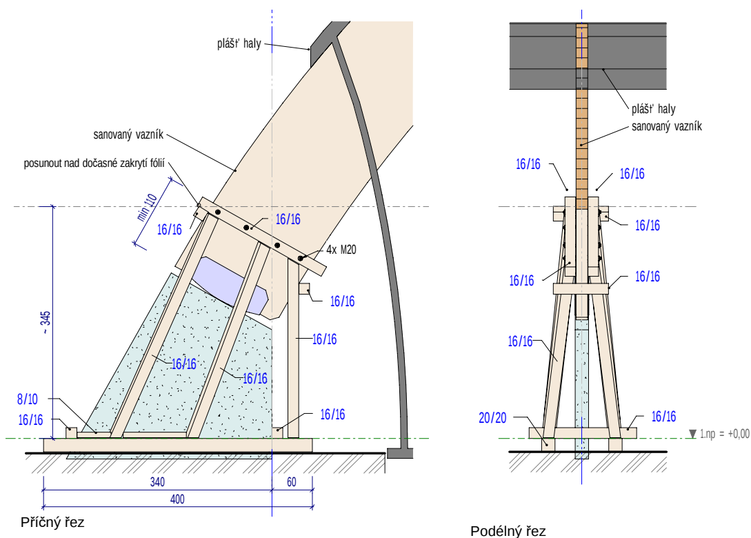
Obrázek 3: Schema dočasného zajištění
