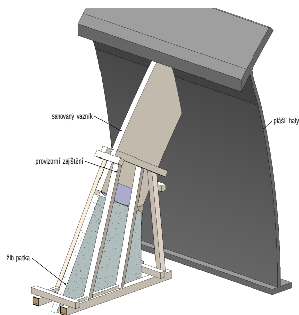
(b) Schema dočasného zajištění
