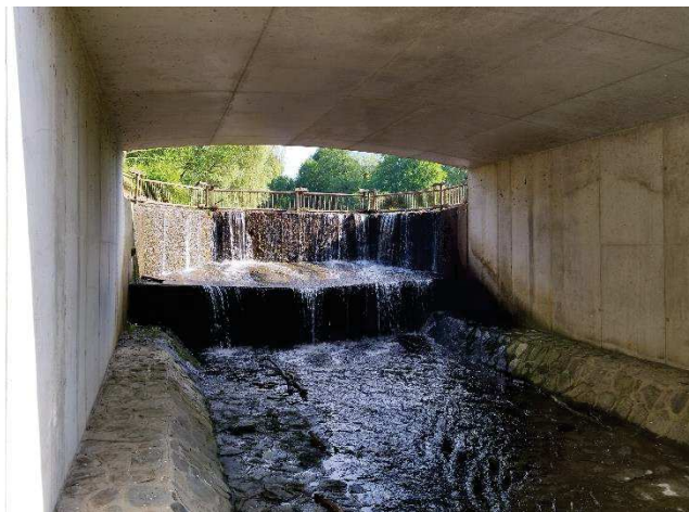
Obr. 2: Bezpečnostní přeliv – průchodnost pro vydru: Neprůchodný BP (vlevo) – svislá přelivná hrana výšky 1 m je nepřekonatelná pro vydru i pro většinu dalších živočichů. Zde je bariérový účinek navíc zvýšen předsazenou ocelovou lávkou s česlemi. Zvířata migrující podél vodního toku jsou nucená přebíhat přes frekventovanou silnici; vpravo - neprůchodný BP z pohledu vydry migrující proti proudu vodního toku. Vydra je v tomto případě schopná projít most pod silnicí, narazí ale na svislou zeď bezpečnostního přelivu, jehož bariérový účinek je navíc zvýšen kovovými česlemi. Zvíře nemá jinou možnost než se vrátit a pokusit se přeběhnout vrchem hráze rybníka s frekventovanou silnicí.
