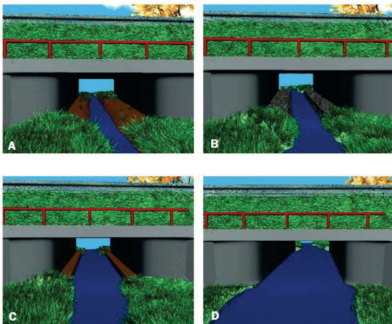
Obr. 51: Různé varianty zajištění suchých břehů pod mostem pro průchod vudry: A - přirozené břehy (optimální situace), B – kamenné postranní bermy (přijatelné řešení), C – zděné či dřevěné postranní lávky (mezí řešení) a most bez suchých břehů v podmostí (neakceptovatelné řešení) (D). Převzato z metodiky Vudra a doprava (Hlaváč a kol., 2017).
