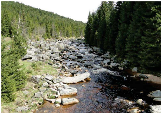
Obr. 14b: Další příklady erozních údolí typu V, zpravidla na horních úsecích toků, ale také v členitých terénech na středních tocích (přírodně bez vyvinuté nivy, bez předpokladu posuzování rozlivu a dalších charakteristik); také v těchto příkladech břehová eroze odpovídá říčnímu vzoru (hydromorfologickému typu vodního toku) – viz parametr 5
