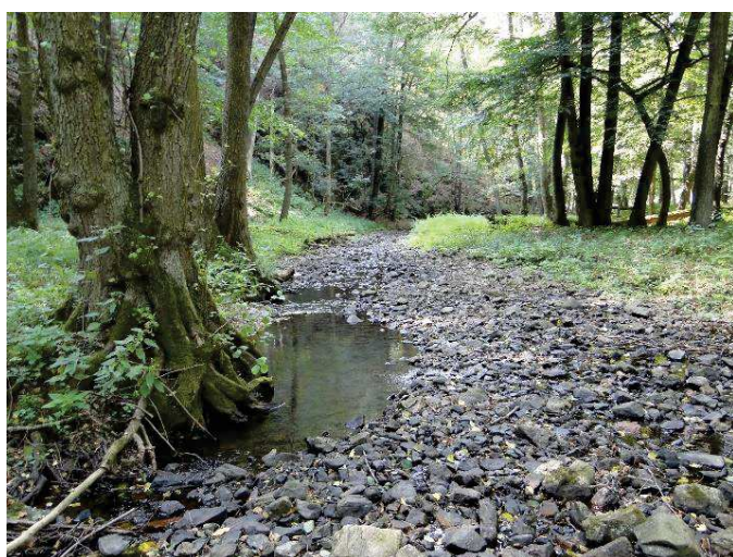
Obr. 15: Neckovité údolí (boční eroze zpravidla zákrutového koryta VT s úzkou nivou omezenou tvarem údolí, střídavě pár metrů prostoru pro rozliv na levém nebo pravém přehu)
