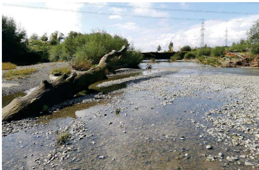
Obr. 62: Štěrkonosné koryto Bečvy – štěrkové lavice a mělčiny
