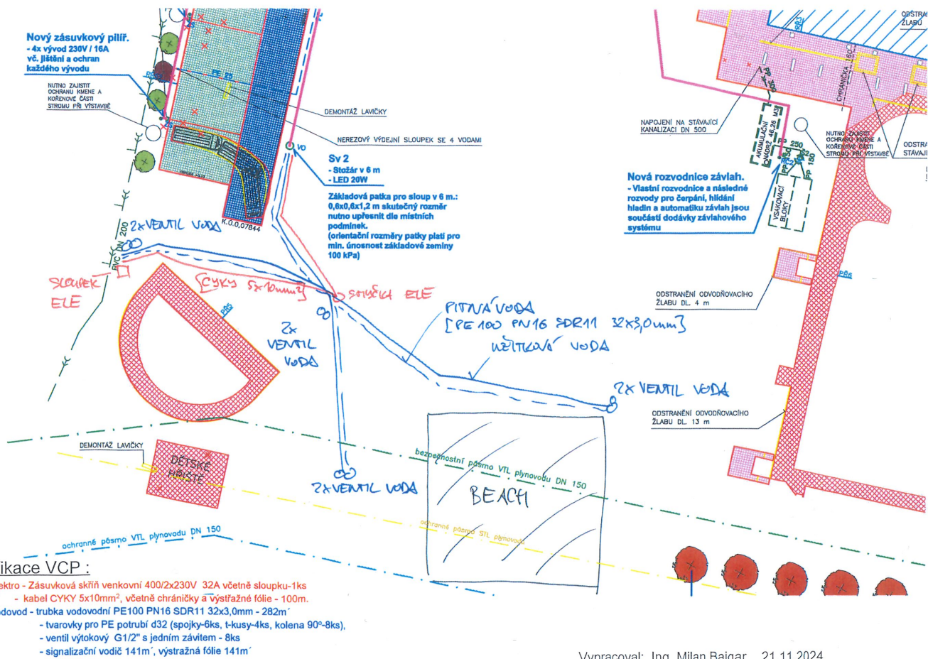
Příloha č.5 k dodatku č.1 - situační výkres - zákres víceprací
