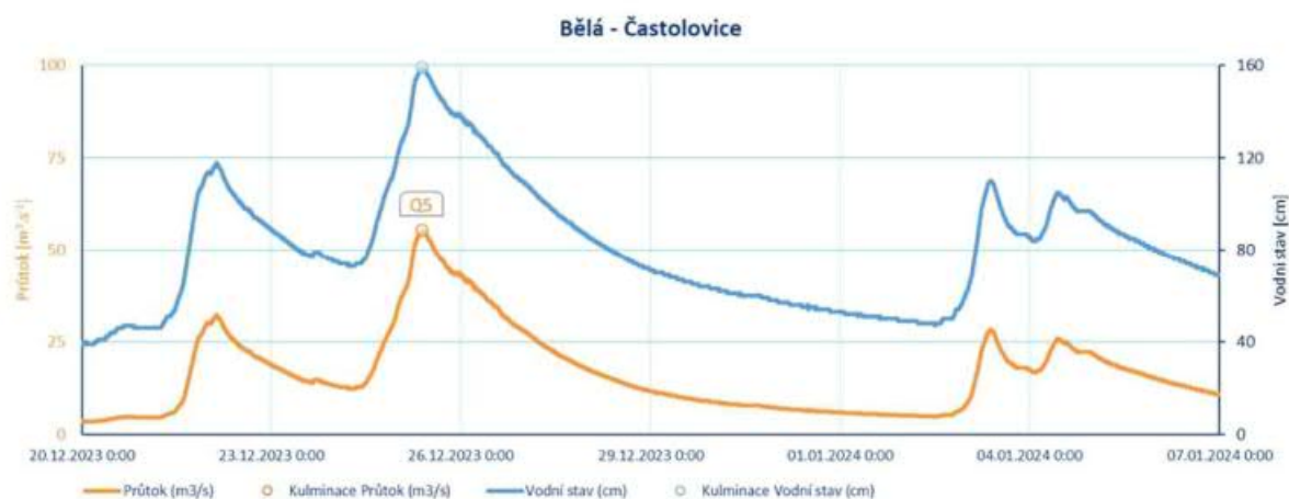
Obr. 11 Průběh průtoků (vodních stavů) na Bělé v profilu Častolovice od 20. 12. 2023 do 7. 1. 2024.
