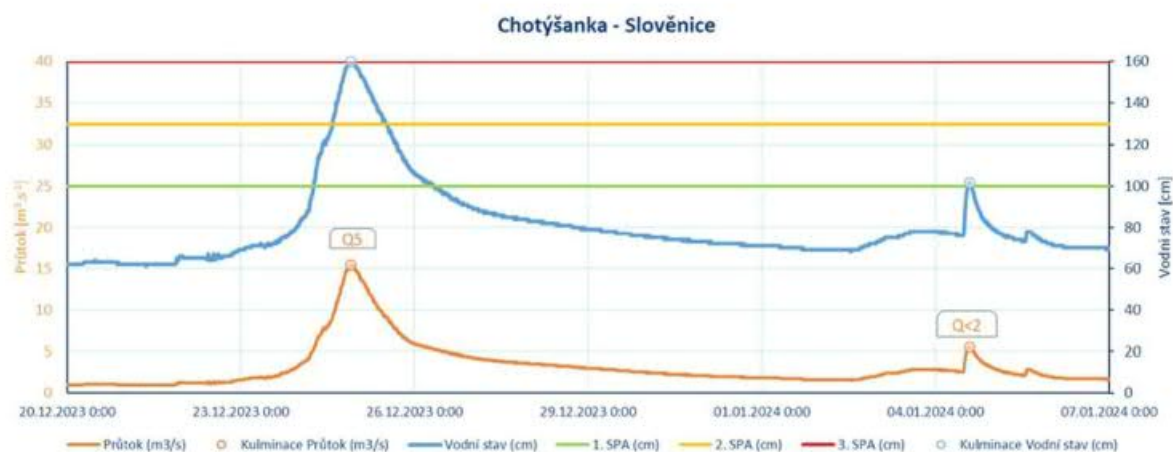
Obr. 28 Průběh průtoků (vodních stavů) na Choýšance v profilu Slověnice od 20. 12. 2023 do 7. 1. 2024.
