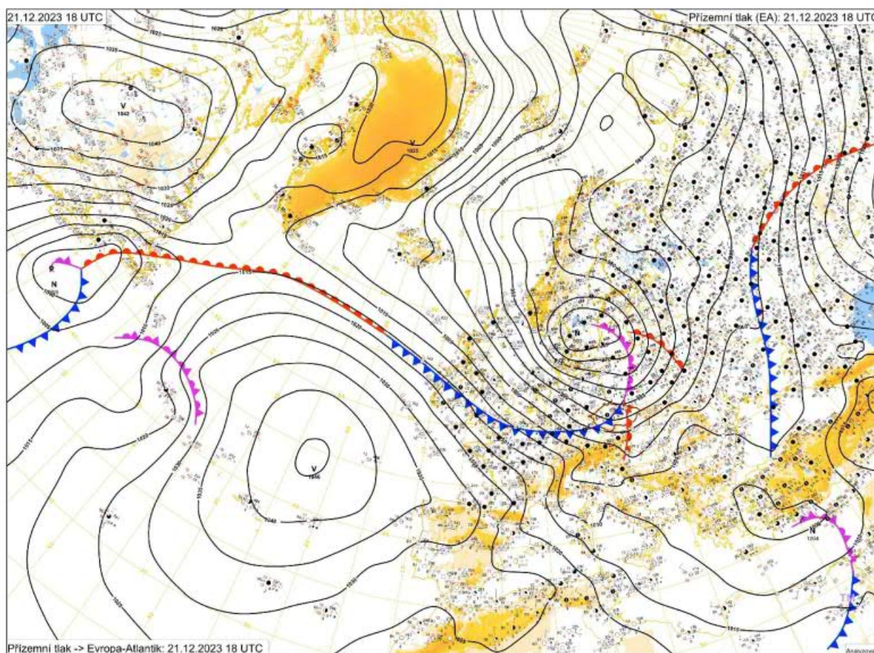
Obr. 1 Přizemní synoptická situace 21. 12. 2023 18 UTC (níže)
