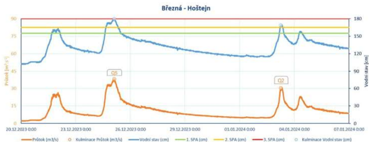
Obr. 38 Průběh průtoků (vodních stavů) na Březné v profilu Hoštejn od 20. 12. 2023 do 7. 1. 2024.
