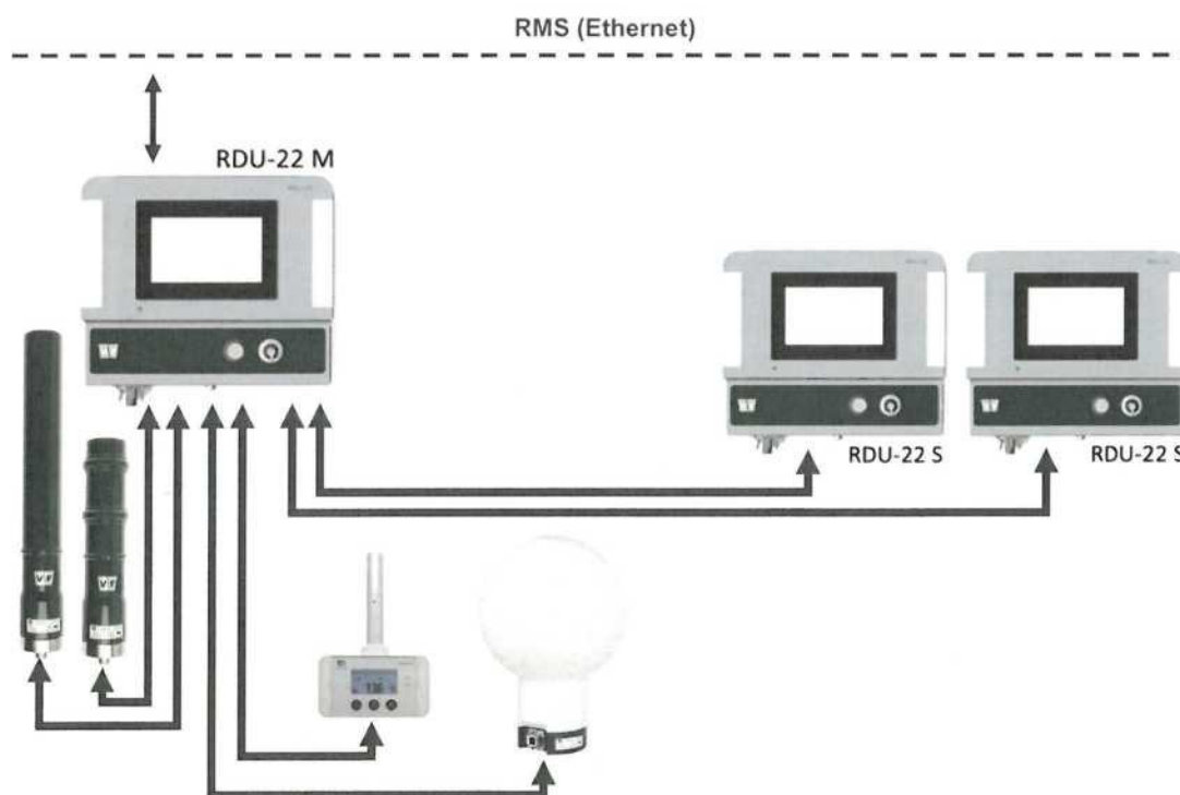
Příklad zapojení RDU-22M s RDU-22S a vybranými detektory do systému RMS
