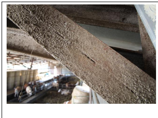
Foto 114 – pohled na ocelovou konstrukci střechy
