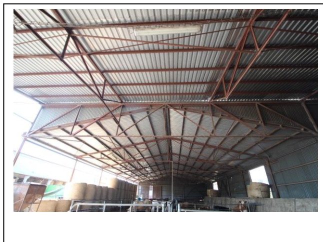
Foto 122 – pohled na ocelovou konstrukci Střechy – štítová stěna
