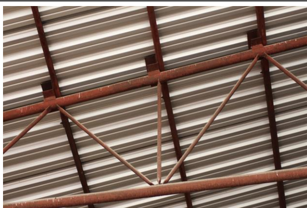
Foto 131 – pohled na ocelovou konstrukci střechy
