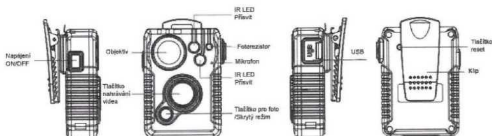
Obrázek 2: Popis kamery PPC 04 Pro
