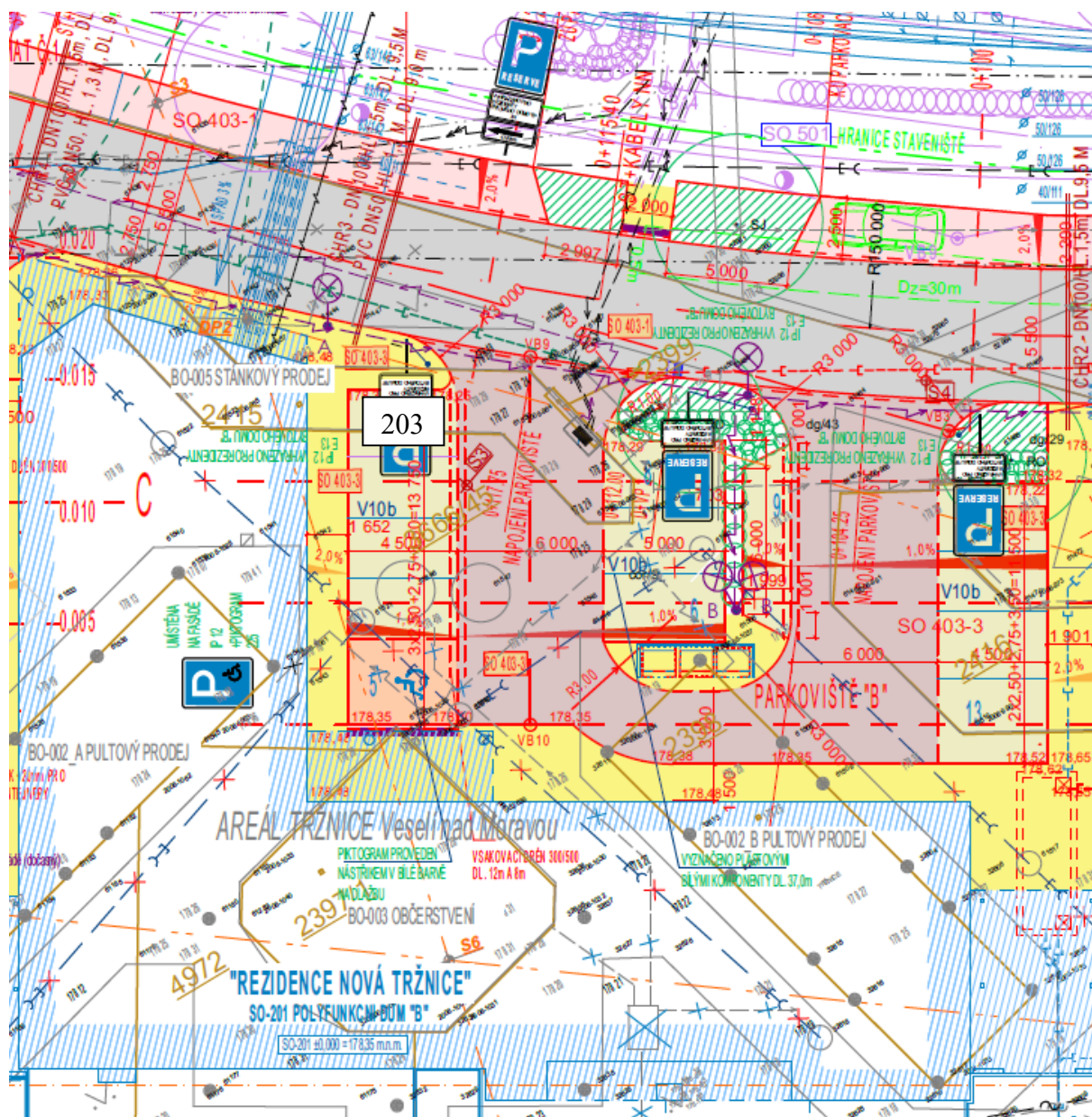
Příloha č. 1: Situační plánec s vyznačením parkovacího místa
