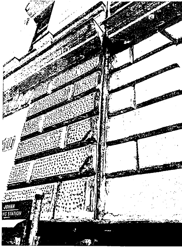
Divadlo pod lampou – poškozené okapové svody, zatékání do fasády
