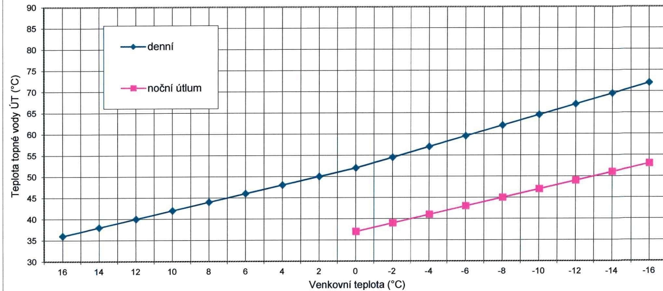
Teplotní křivka
