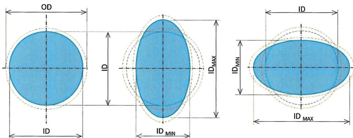
Znázornění vnitřního průměru, vnějšího průměru a parametrů pro stanovení deformace, resp. ovality
