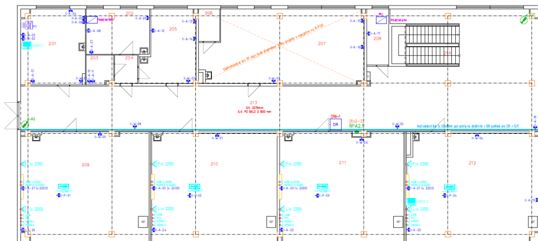
PŮDORYS 3.NP (M 1:100)
